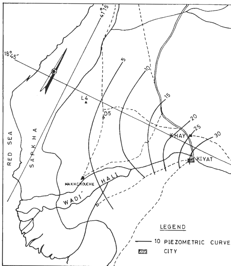
FIG. 9. Piezometric surface map of Wadi Hali.
