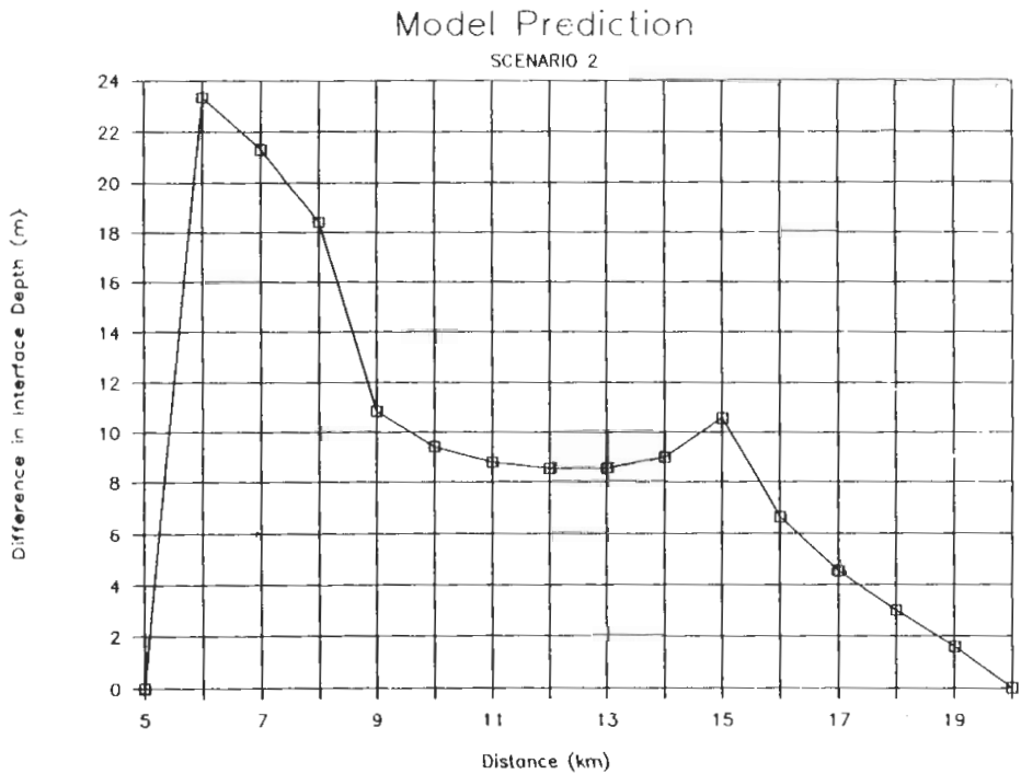
FIG. 18. Rise in interface depth (Scenario 2).
