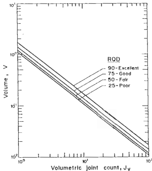
FIG. 5. Bar block RQD-J v -V charts.
