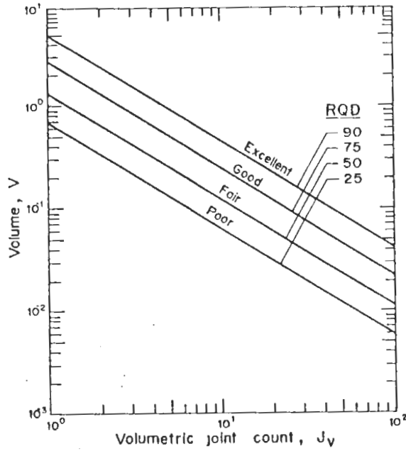
FIG. 11. Plate block RQD-J_v-V charts, ( \alpha = 0.1 ).
