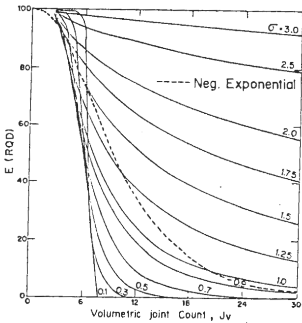
FIG. 4. Bar block RQD-J_v charts, ( t = 0.20 m).
