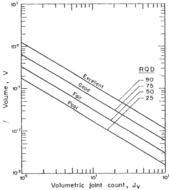
FIG. 12. Plate block RQD-J_v-V charts, ( \alpha = 0.5 ).
