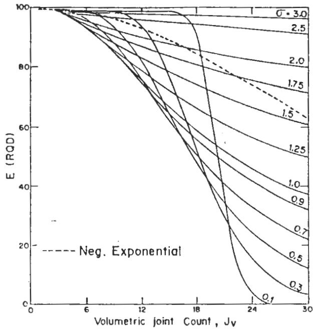
FIG. 3. Bar block RQD-J_v charts, ( t = 0.05 m).
