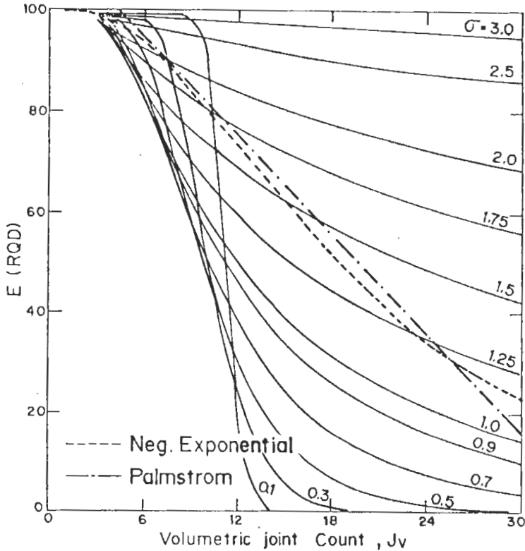
FIG. 2. Bar block RQD-J_v charts, ( t = 0.10 m).
