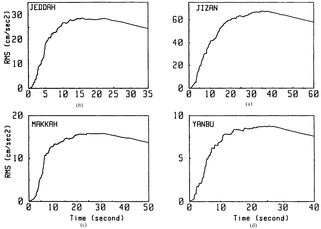
FIG. 10. Root-mean-square acceleration integral: a) Jizhan, b) Jeddah, c) Makkah, d) Yanbu.
